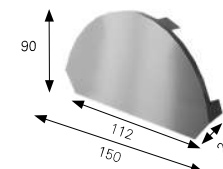
VÉGLEMEZ FÉLKÖRÍVES GERINCLEMEZHEZ
