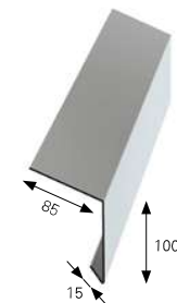
FELSŐ ERESZSZEGÉLY
