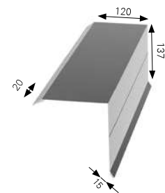
OROMDESZKA SZEGÉLY I
