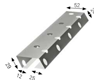
UNIVERZÁLIS SZELLŐZTETŐ BÁDOGOS ELEM
