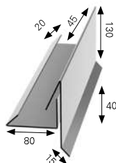
OROMDESZKA SZEGÉLY II
