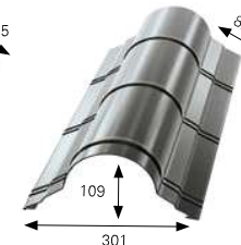
FÉLKÖRÍVES GERINCLEMEZ SZÉLES
