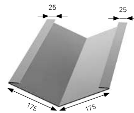
VÁPASZEGÉLY
