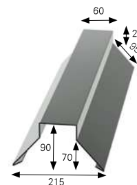
TRAPÉZ GERINCLEMEZ
