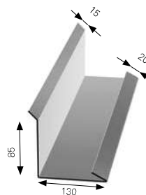
FALSZEGÉLY II
