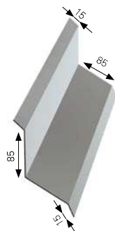
FALSZEGÉLY I
